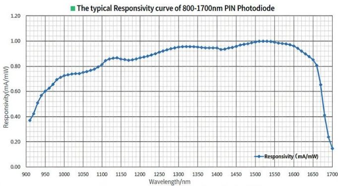
响应曲线
